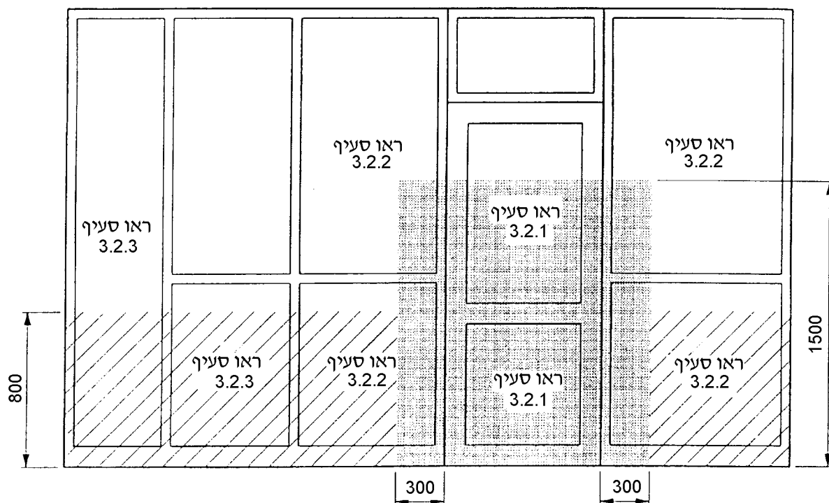
ציור 1 - אזורי סכנה (המידות במילימטרים)
